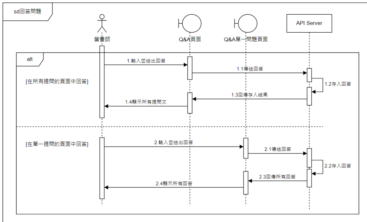
▲圖 6-1-16 回答問題之循序圖
