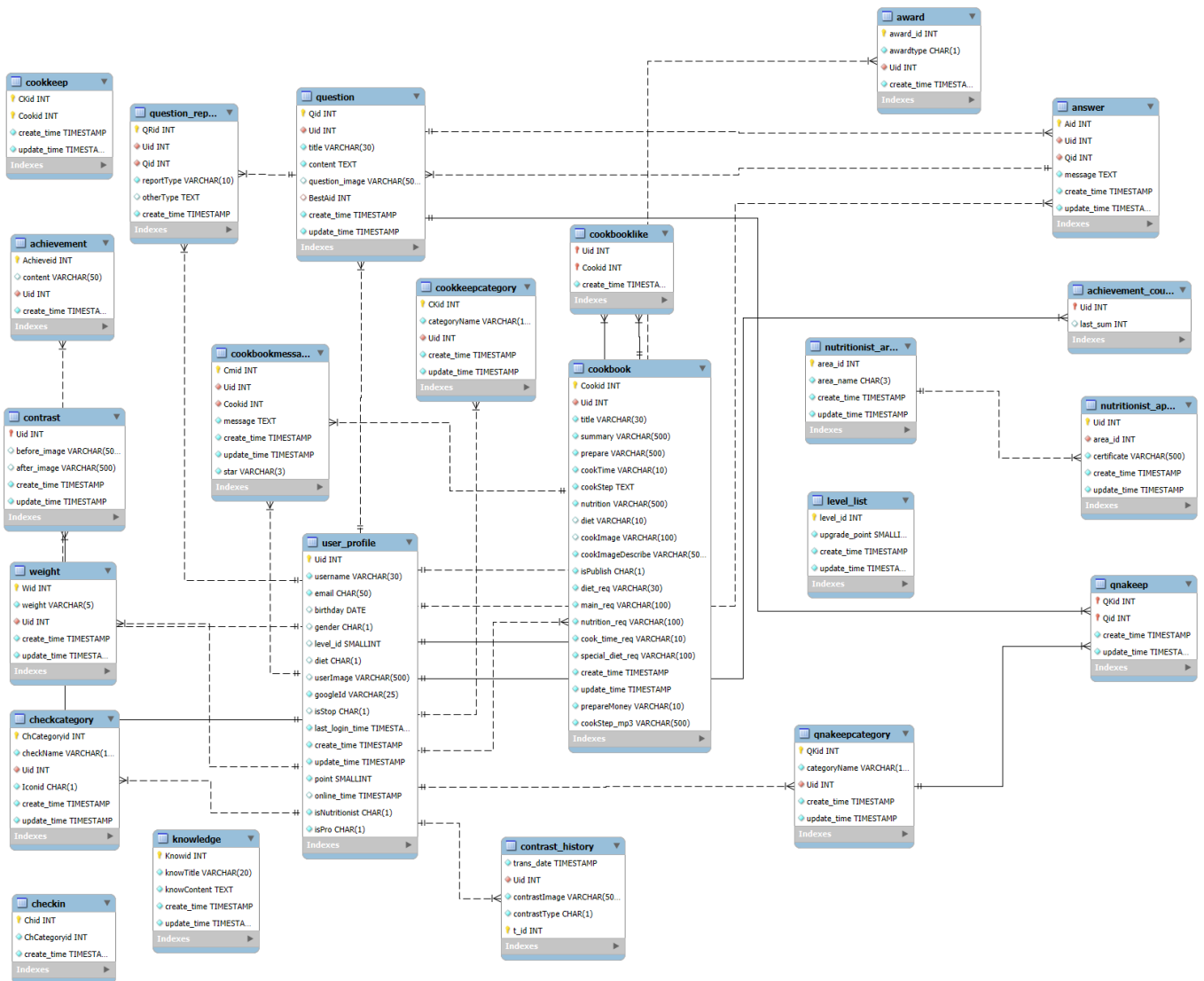
▲圖 8-1-1 資料庫關聯圖
