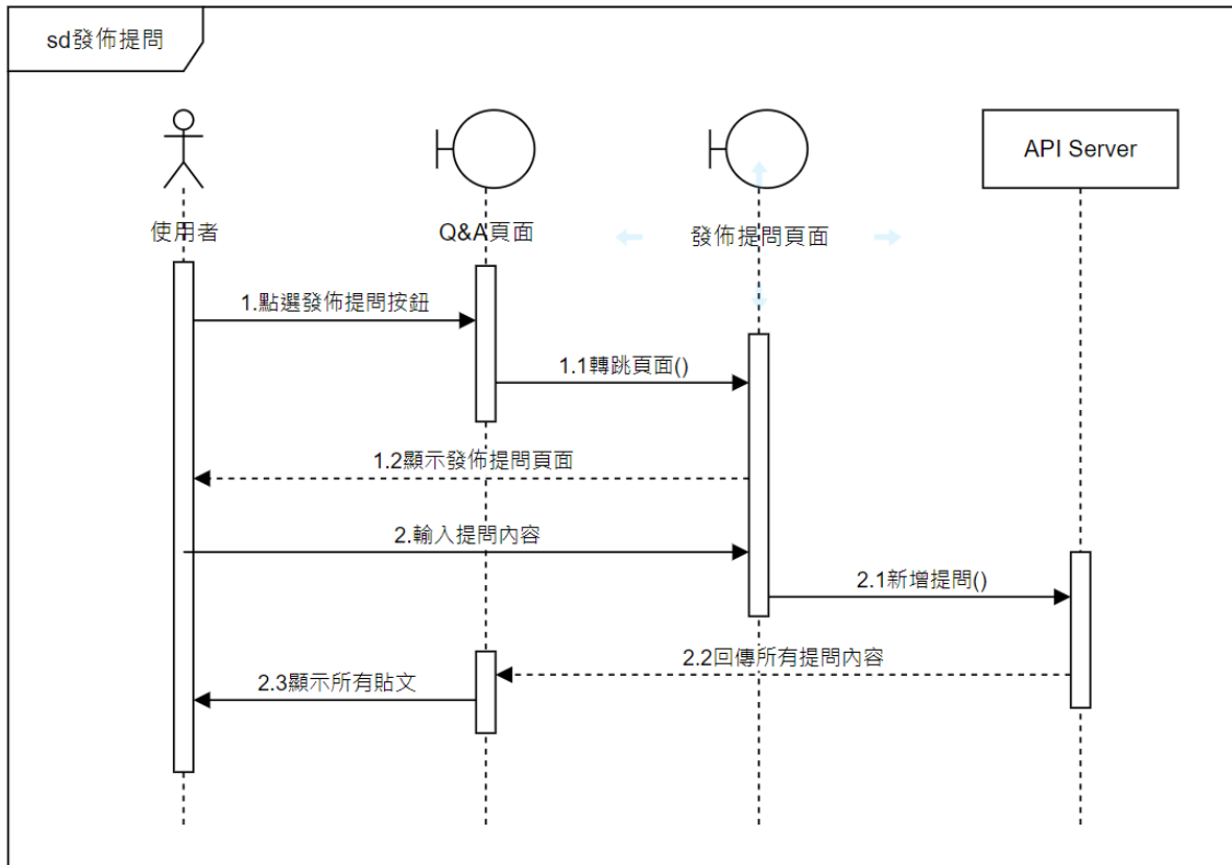
▲圖 6-1-14 發佈提問之循序圖
