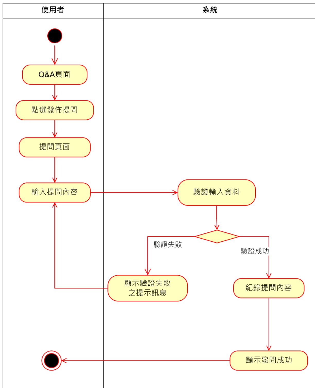
▲圖 5-2-14 活動圖之發佈提問
