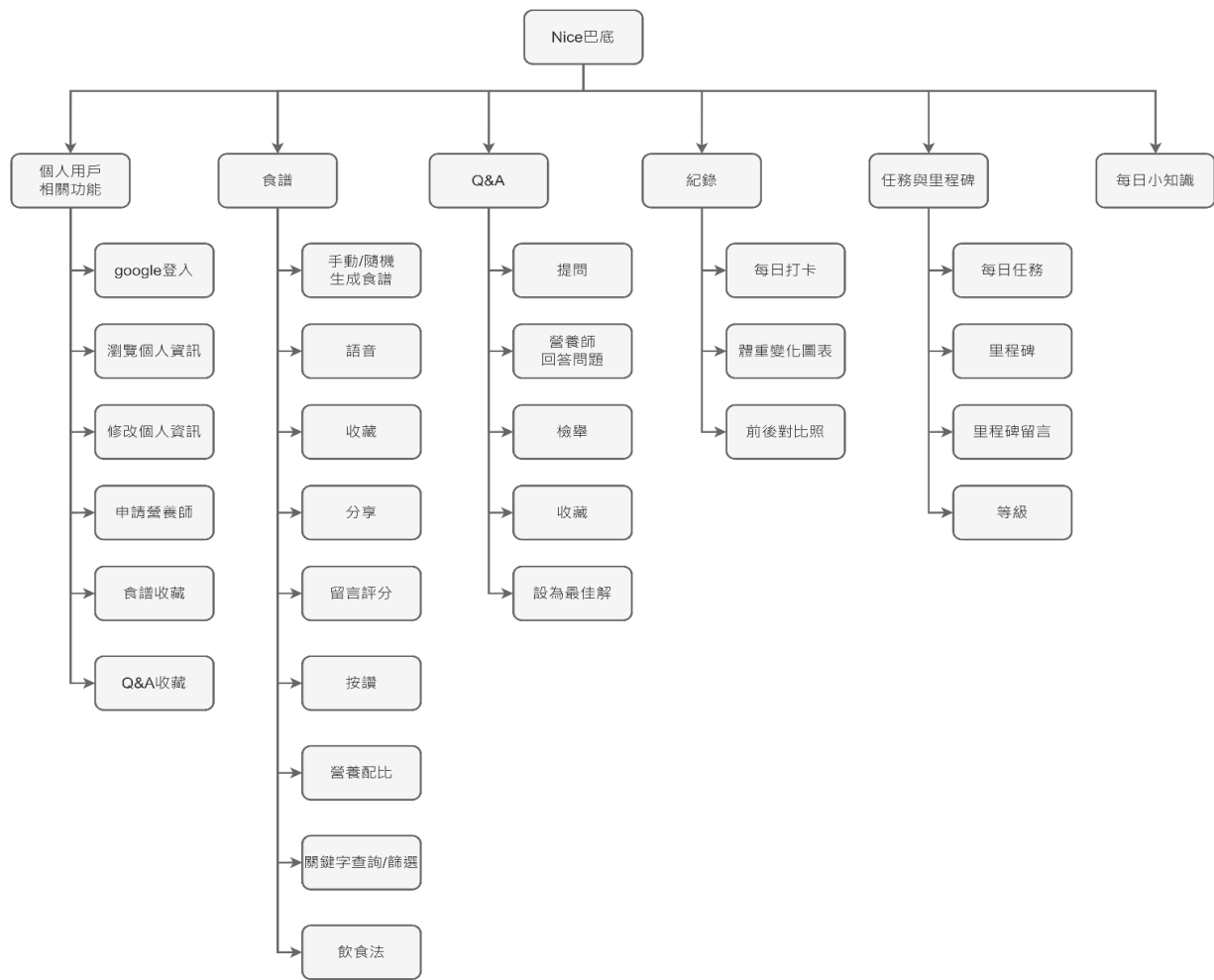
▲圖 3-1-2 系統功能架構圖
