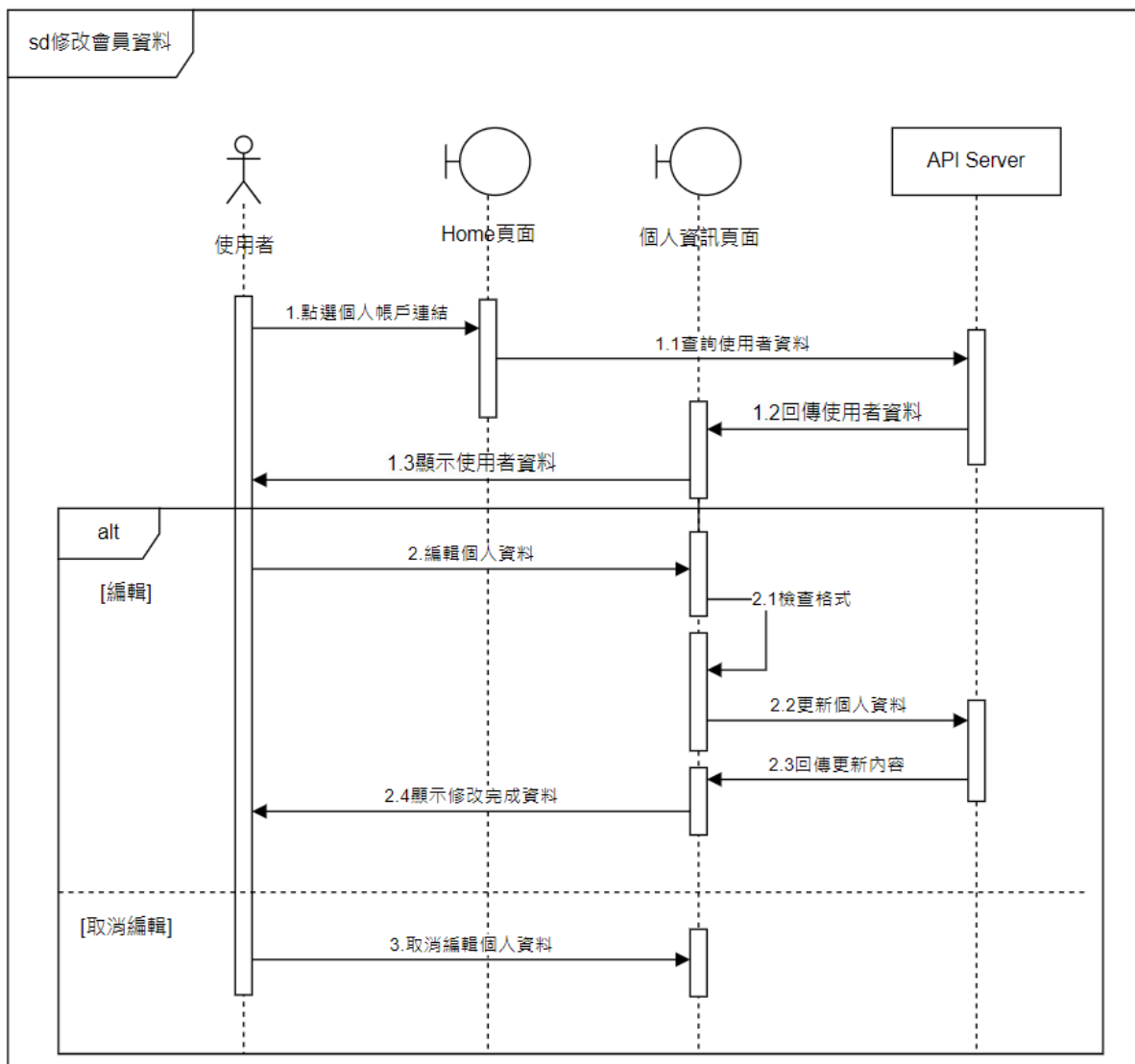
▲圖 6-1-3 修改會員資料之循序圖
