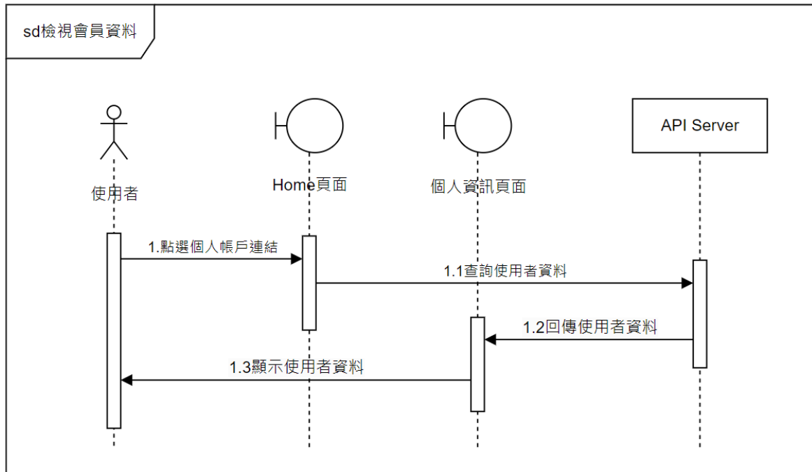
▲圖 6-1-2 檢視會員資料之循序圖
