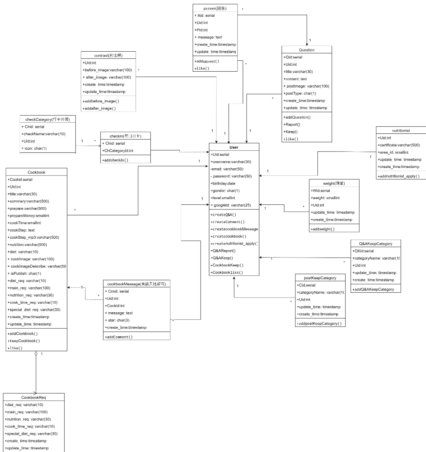
▲圖 5-3-1 分析類別圖
