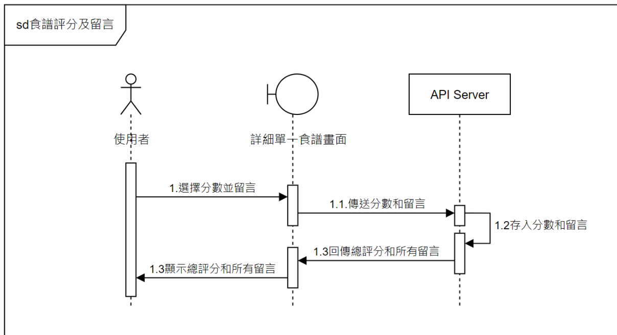
▲圖 6-1-8 食譜評分及留言之循序圖
