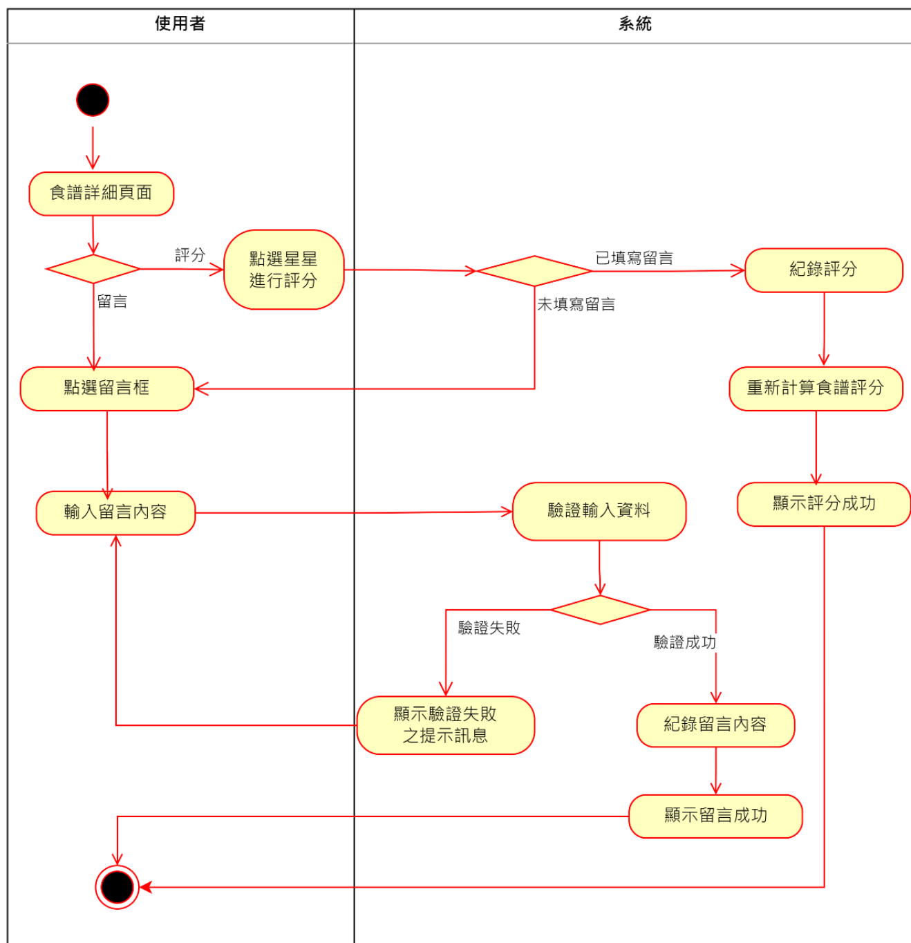
▲圖 5-2-7 活動圖之食譜評分及留言
