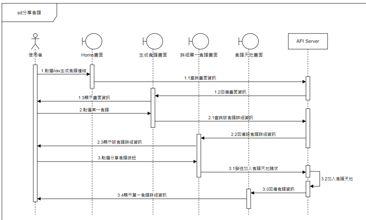
▲圖 6-1-7 分享食譜之循序圖
