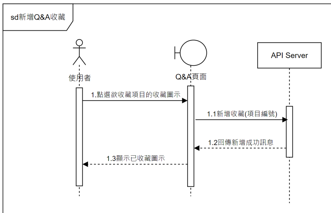
▲圖 6-1-13 新增 Q&A 收藏之循序圖
