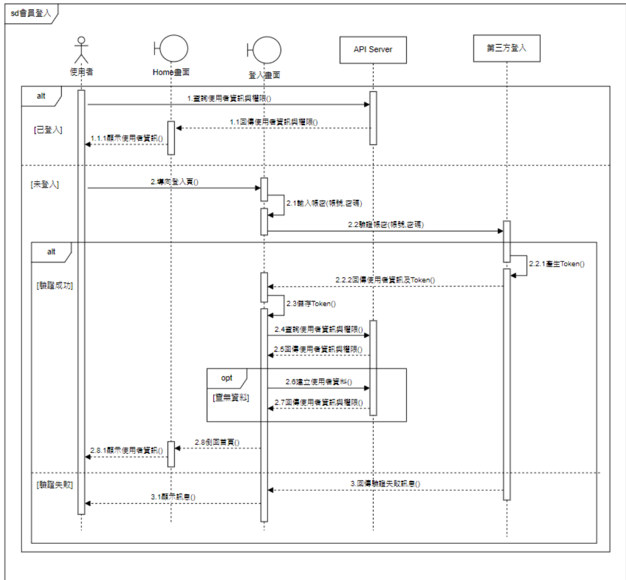
▲圖 6-1-1 登入之循序圖
