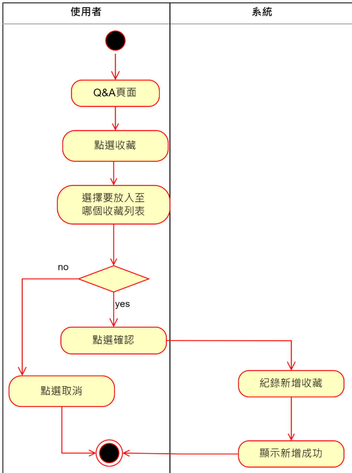
▲圖 5-2-12 活動圖之新增 Q&A 收藏
