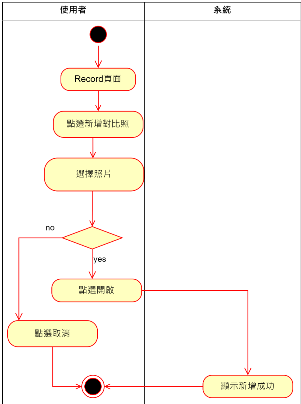
▲圖 5-2-17 活動圖之新增前後對比照
