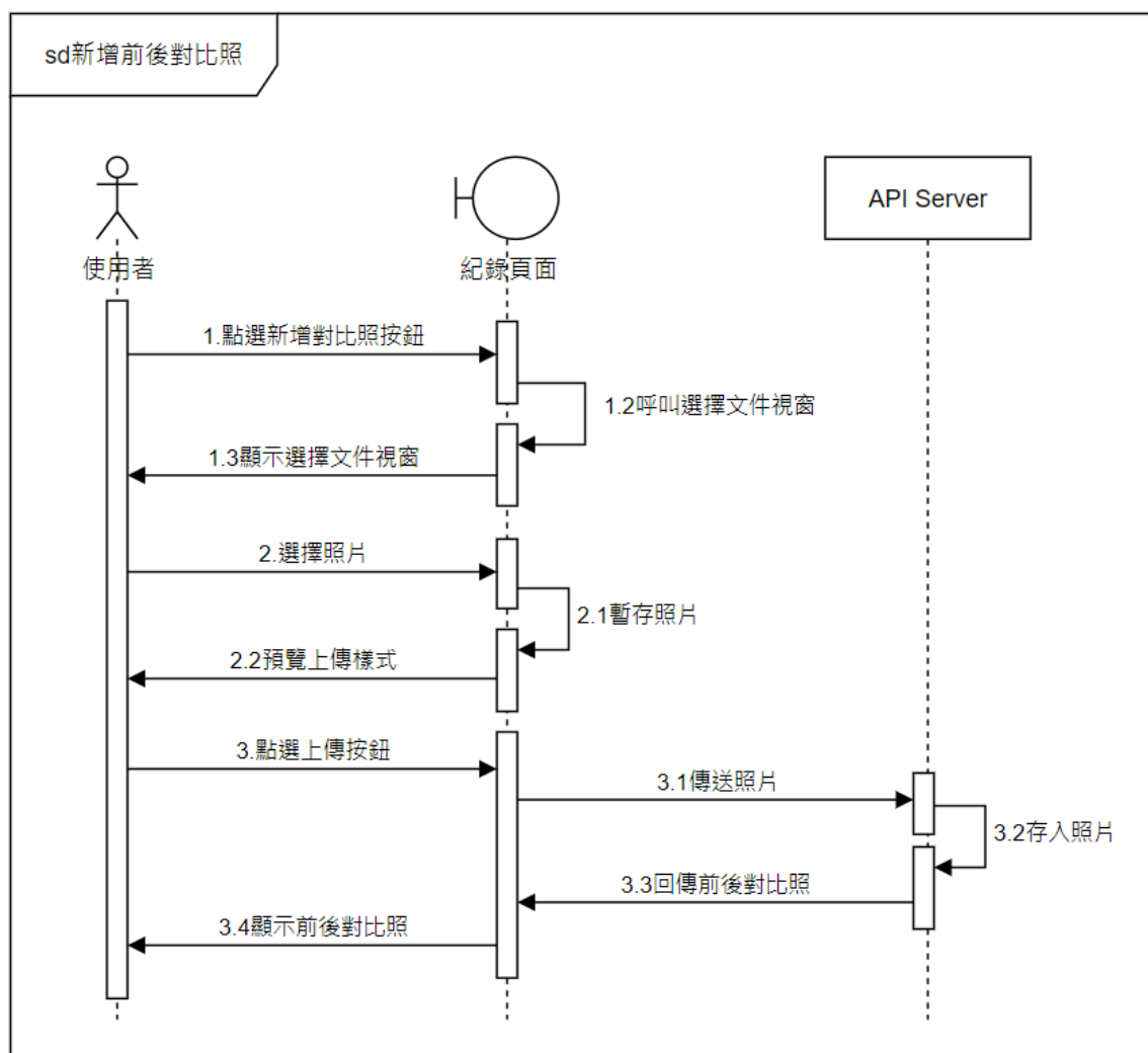
▲圖 6-1-19 新增前後對比照之循序圖
