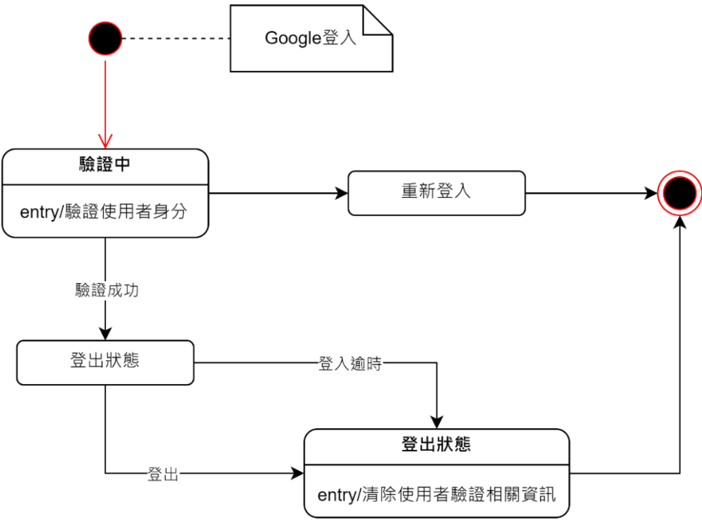
▲圖 7-4-1 登入之狀態機圖
