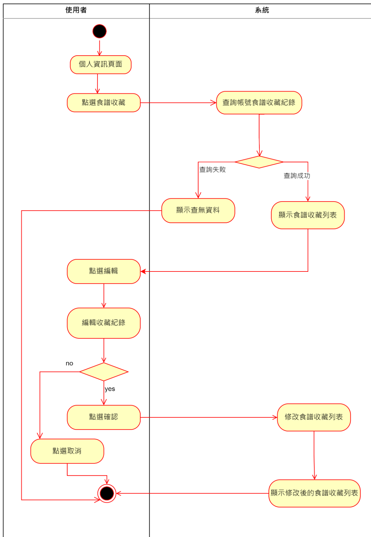
▲圖 5-2-10 活動圖之修改食譜收藏分類
