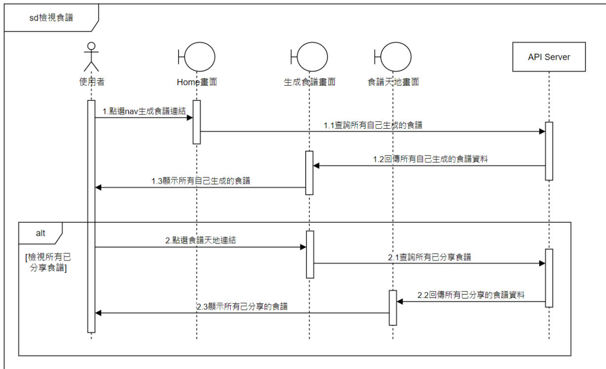
▲圖 6-1-6 檢視食譜之循序圖
