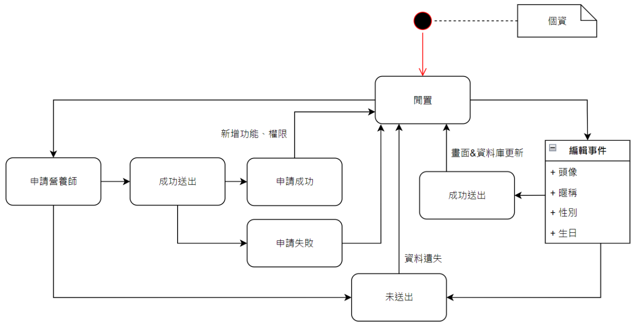
▲圖 7-4-5 個資之狀態機圖
