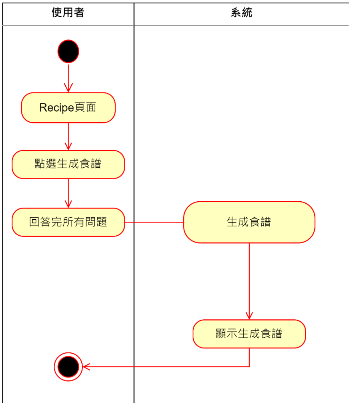
▲圖 5-2-4 活動圖之生成食譜
