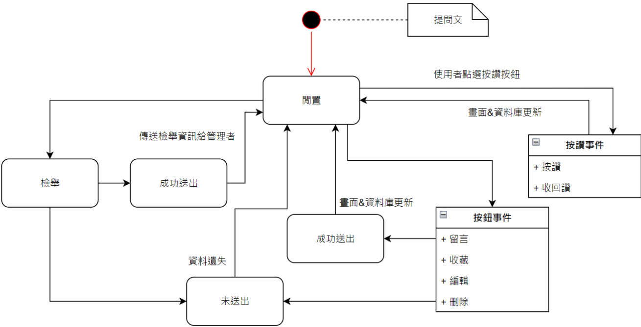
▲圖 7-4-2 提問文之狀態機圖
