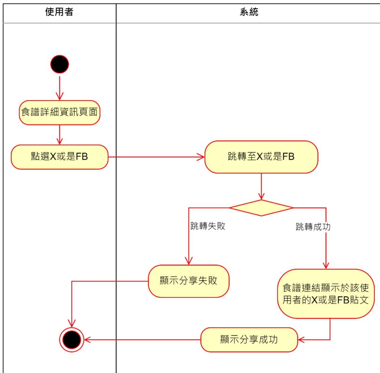
▲圖 5-2-6 活動圖之分享食譜
