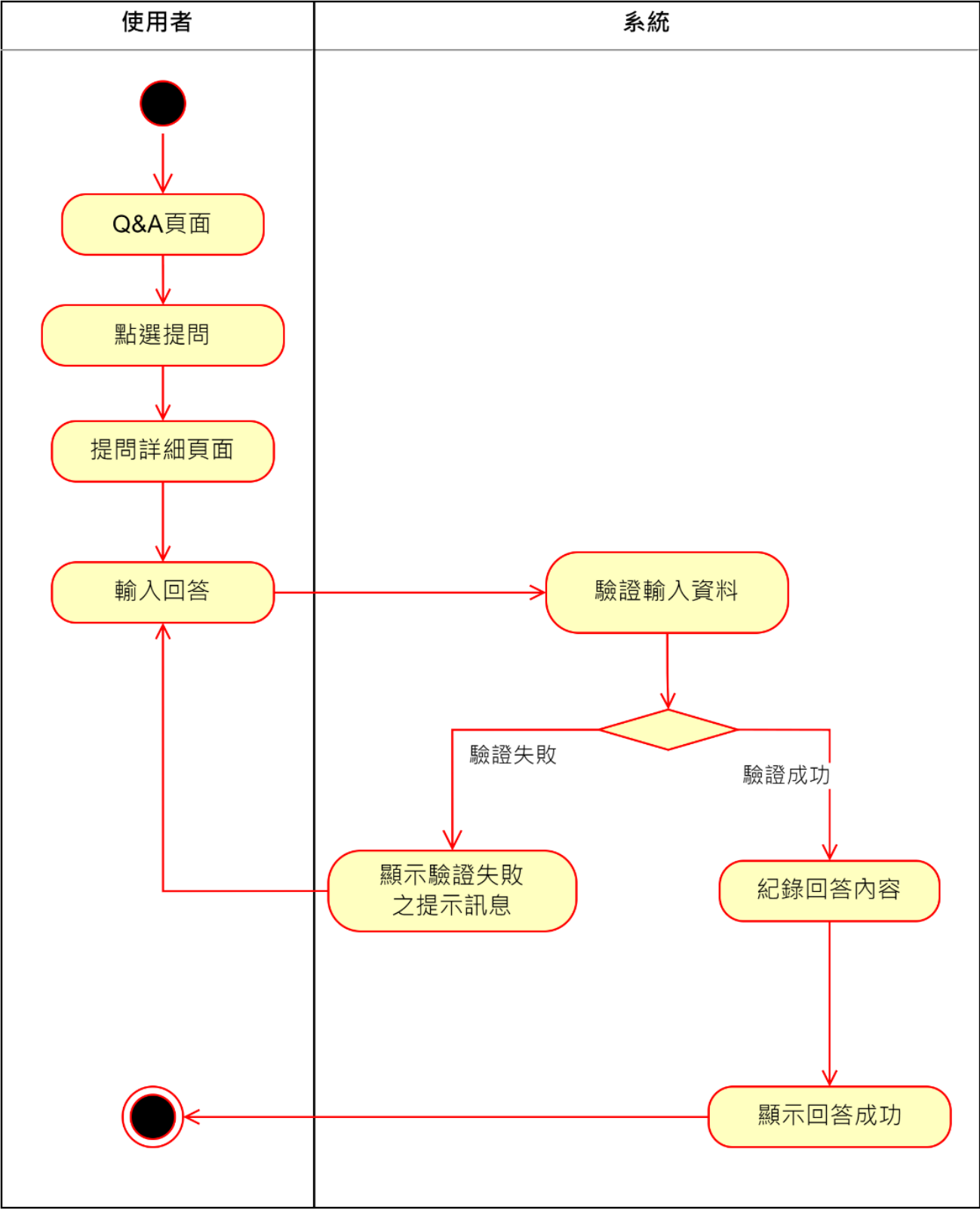
▲圖 5-2-19 活動圖之回答問題
