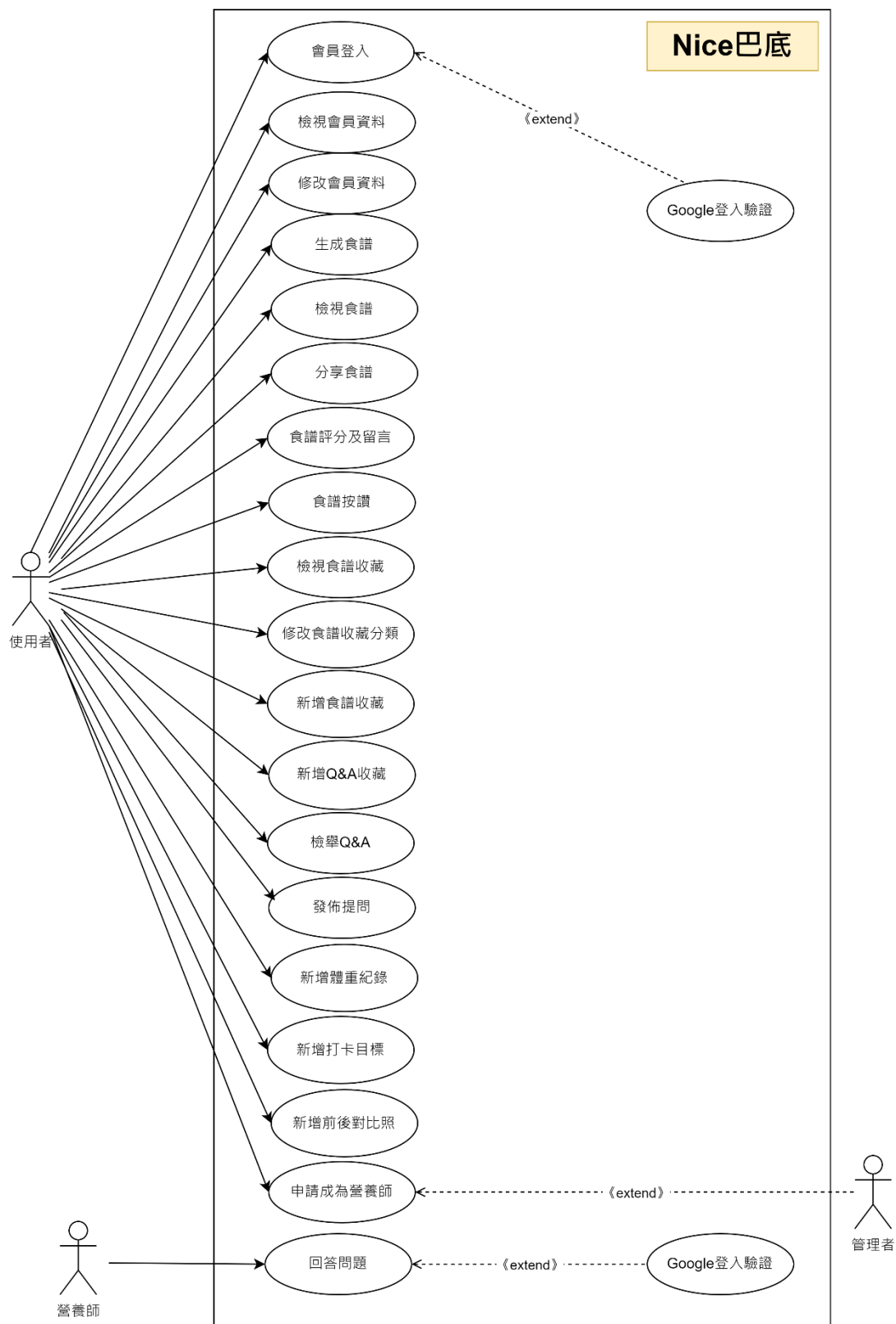
▲圖 5-1-1 使用個案圖
