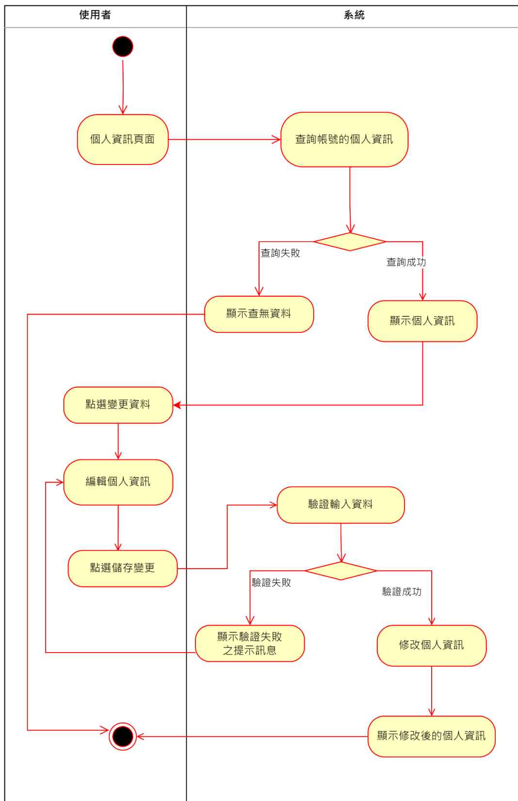
▲圖 5-2-3 活動圖之修改會員資料
