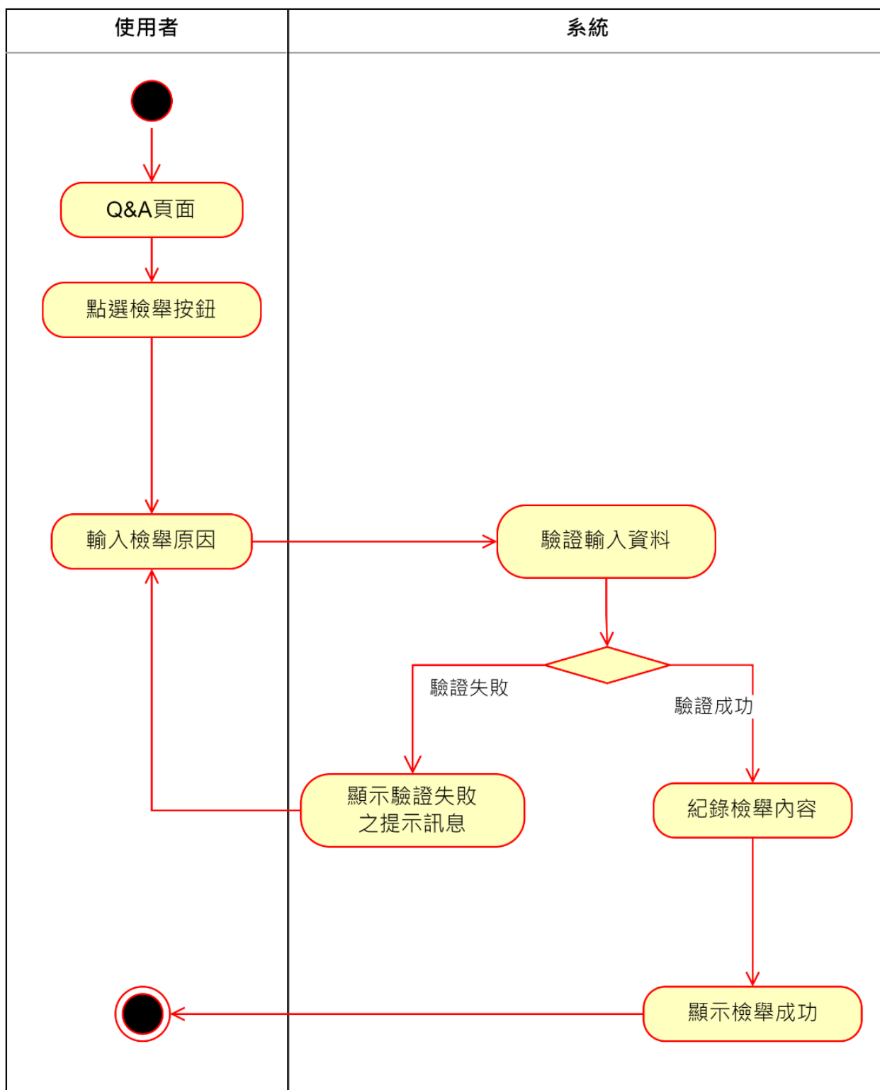
▲圖 5-2-13 活動圖之檢舉 Q&A
