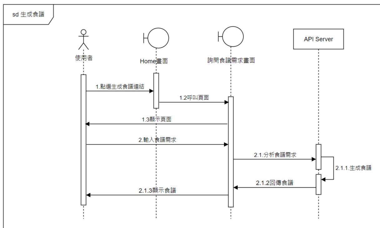
▲圖 6-1-5 生成食譜之循序圖
