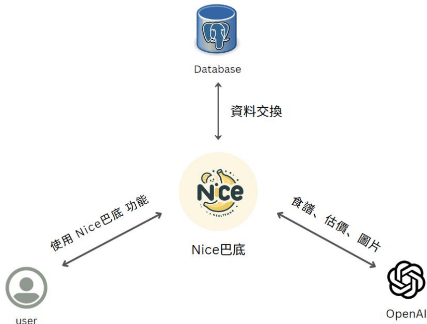
▲圖 3-1-1 系統架構圖
