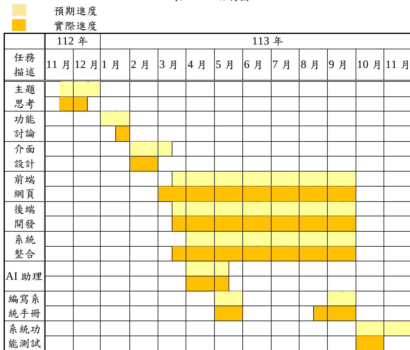
▼表 4-1-1 甘特圖
