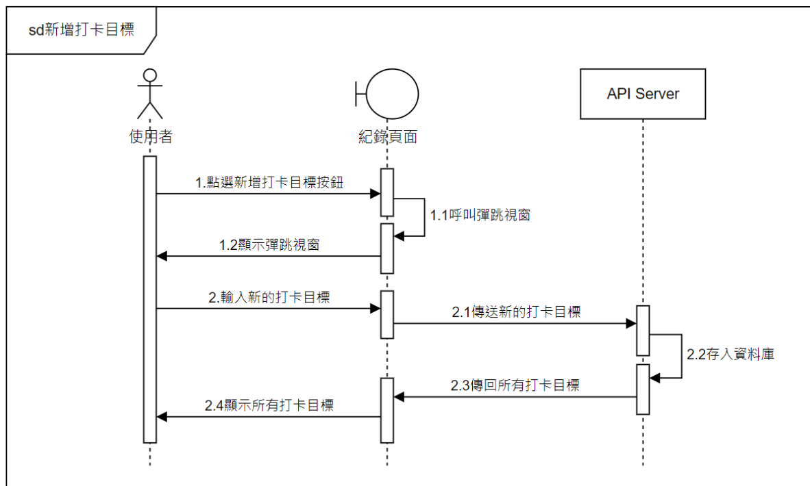
▲圖 6-1-18 新增打卡目標之循序圖
